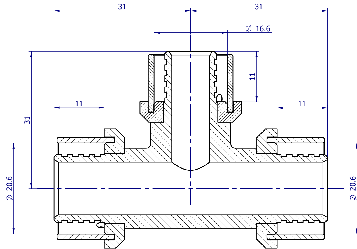
SECTION A-A
