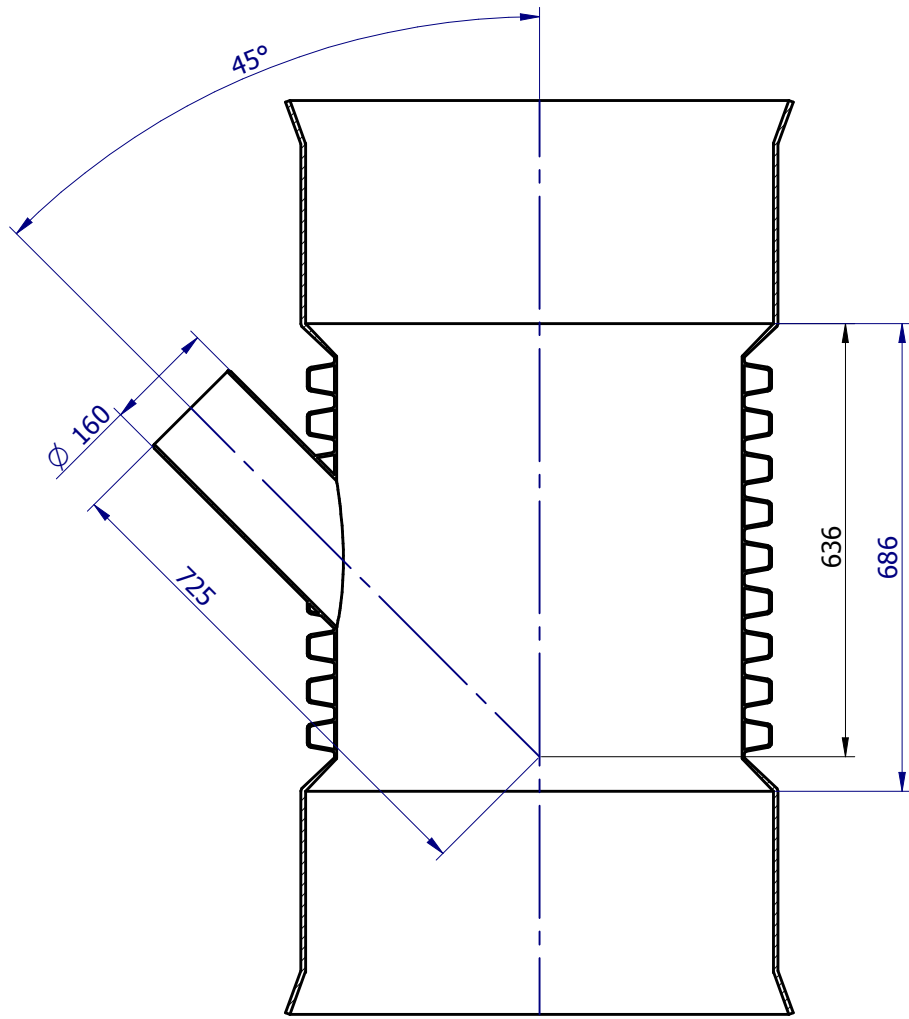
SECTION A-A
