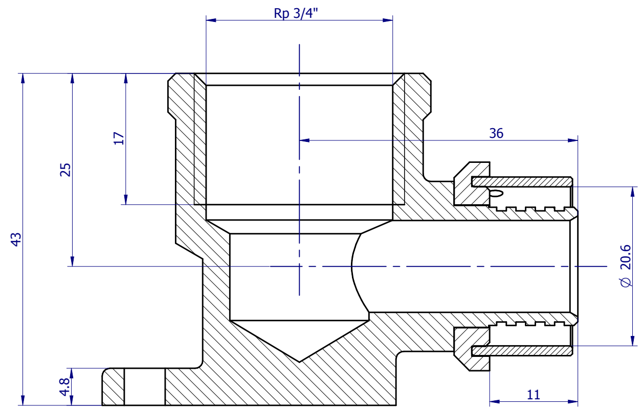
SECTION A-A
