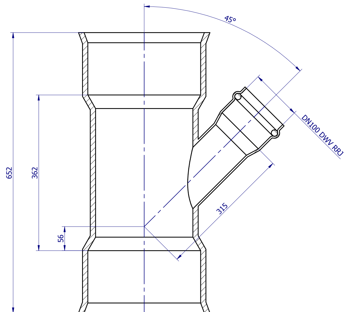
SECTION A-A
